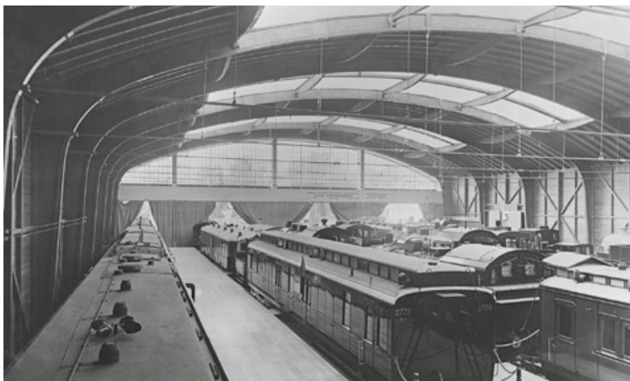
Eisenbahnalle für die Weltausstellung in Brüssel von Architekt Peter Behrens. Das Tragwerk bilden Rahmenkonstruktionen aus mit Kaseinklebstoff geklebtem Brettschichtholz. Mit der Entwicklung von Kunstharzklebstoffen ab Mitte der 1930er Jahre wurden neue materialsparende geklebte Konstruktionen entwickelt.
