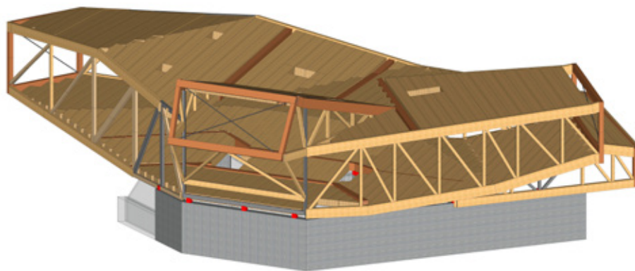
Der Konferenzsaal der Weltorganisation für geistiges Eigentum, kurz WIPO oder OMPI, ist ein höchst unsymmetrisches Gebilde mit weit auskragenden Gebäudeteilen. Das Bauwerk besteht aus Brettschichtholz-Hohlkästen für Boden, Decken und Wände sowie Fachwerkträgern.
