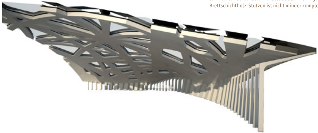
Perspektivischer Schnitt durch das Elefantenhaus in Zürich mit einem siebenteiligen Holz-Verbund-Querschnitt als Dachschale. Die Fassade aus L-förmigen Brettschichtholz-Stützen ist nicht minder komplex.
