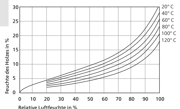
Abb. 2.1 Gleichgewichtsfeuchten von Nadelholz in Abhängigkeit der relativen Luftfeuchte und der Temperatur (nach [11])
