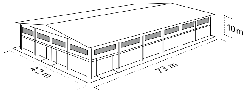
Abb. 3: Hallenabmessungen
