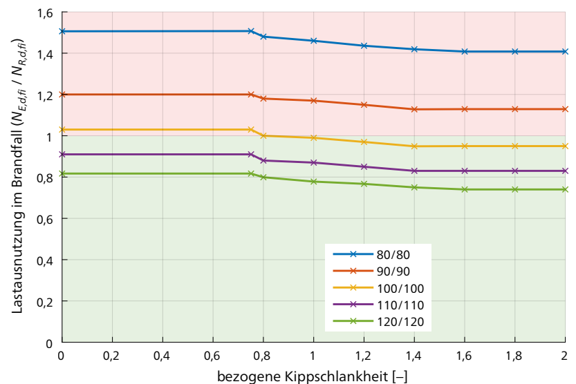
Abb. 12: Lastausnutzung im Brand für verschiedene Querschnitte in Abhängigkeit der bezogenen Kippschlankheit
