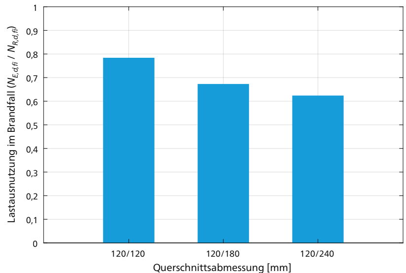
Abb. 11: Lastausnutzung im Brand nach 15-minütiger ETK-Beanspruchung bei Vollauslastung unter Normaltemperatur für verschiedene Biegestäbe
